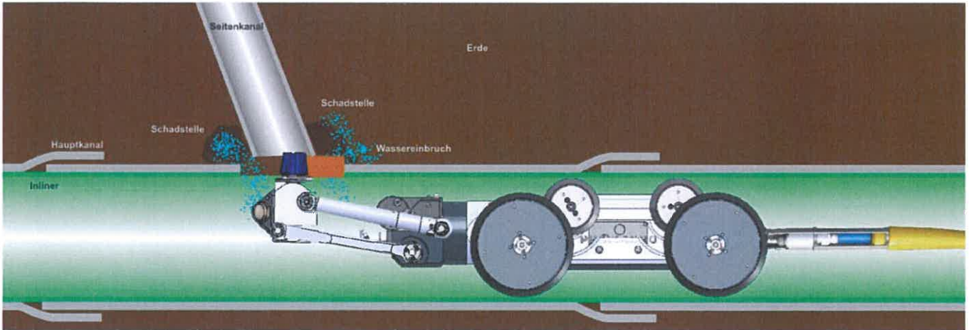
Bild 4. Hinterfräsen der Schlauchlinerkante (entfällt, wenn keine vorherige Sanierung des Hauptkanals mittels Schlauchliner o. Ä. erfolgte)
