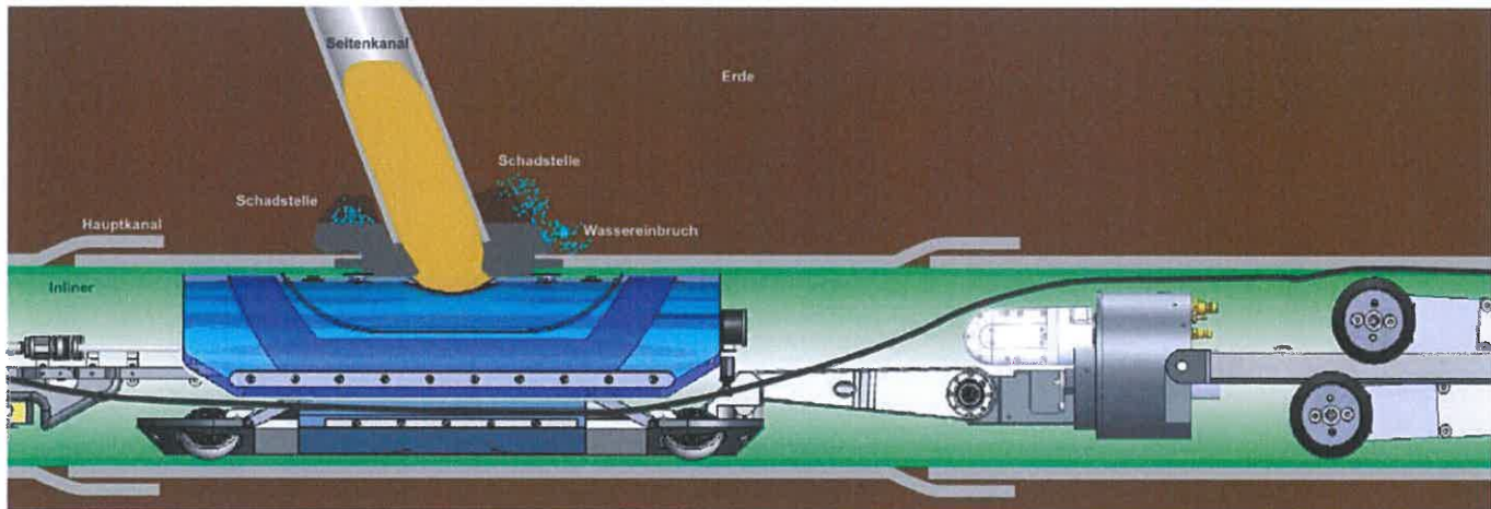
Bild 8. Aufrechterhalten des Anpressdrucks von Schalungsschild und Zulaufblase während der Härtungsphase
