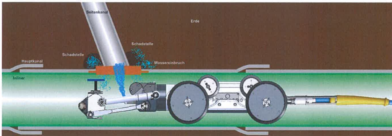
Bild 6. Positionieren des Roboters und aufstellen der Seitenzulaufblase
